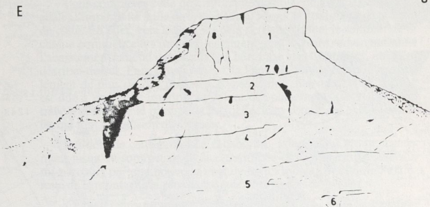
Géologie de la face Nord du Granier
